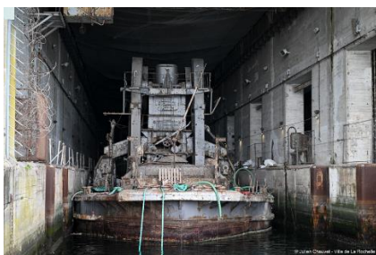
Déplacement de la drague TD6 vers la forme de radoub n°2 du Grand port maritime de La Rochelle © Julien Chauvet
